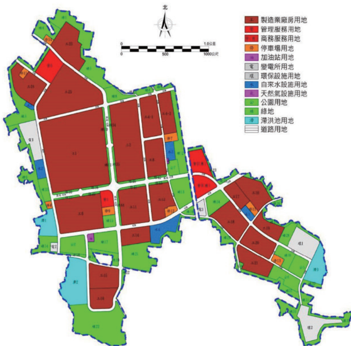
圖 3 高雄園區細部計畫圖 (六變) 108.1.9 發布實施
